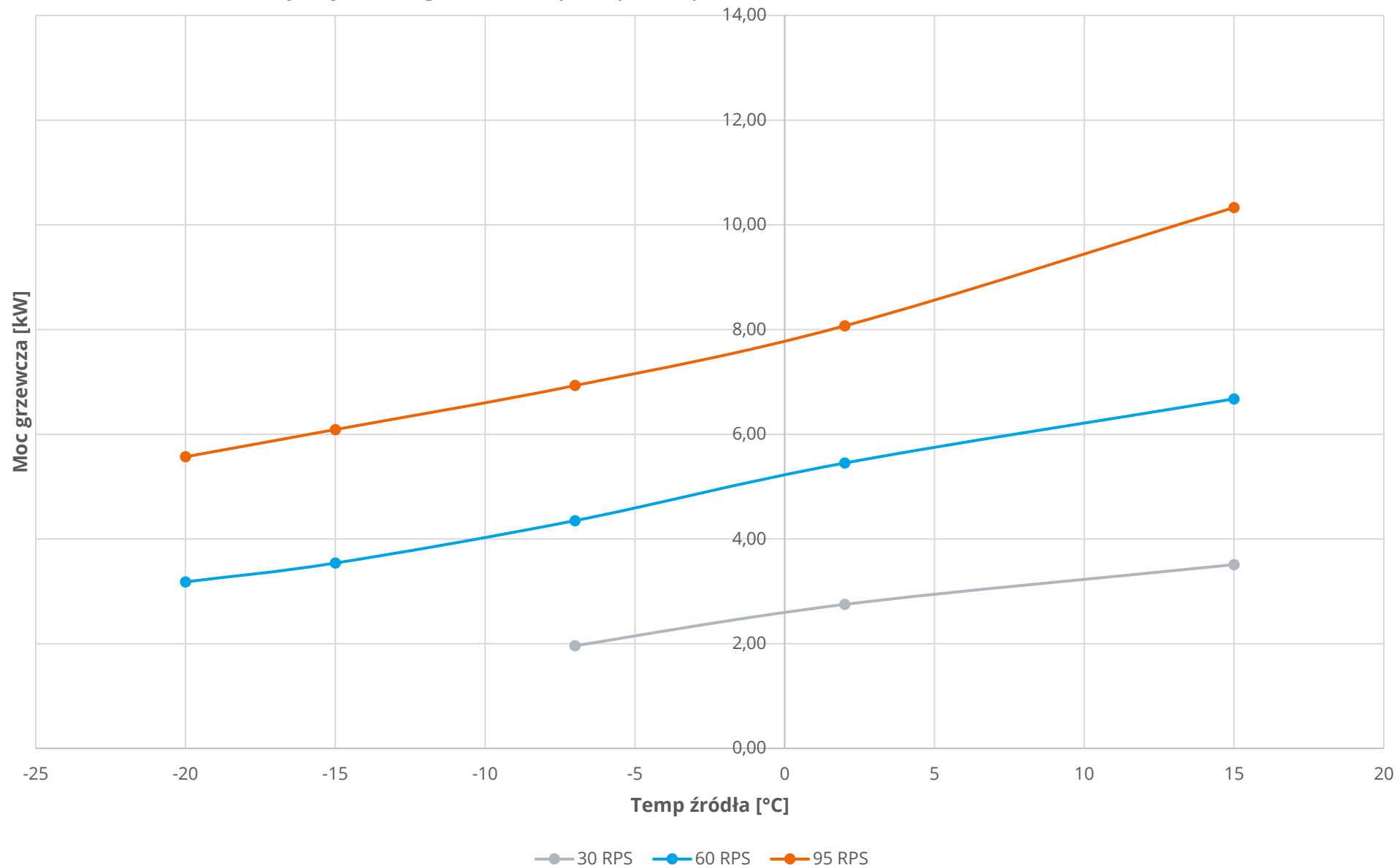
Wydajność ogrzewania pompa ciepła ZHHS-10K, Woda 47/55°C
