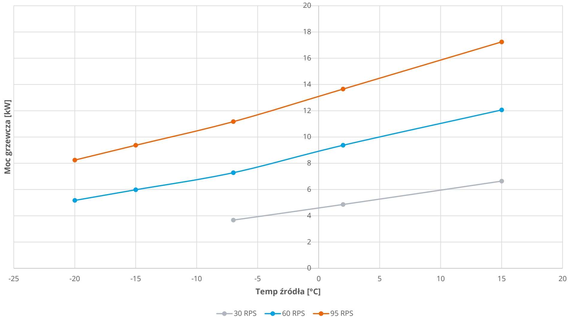
Wydajność ogrzewania pompa ciepła ZHHS-15K, Woda 30/35°C
