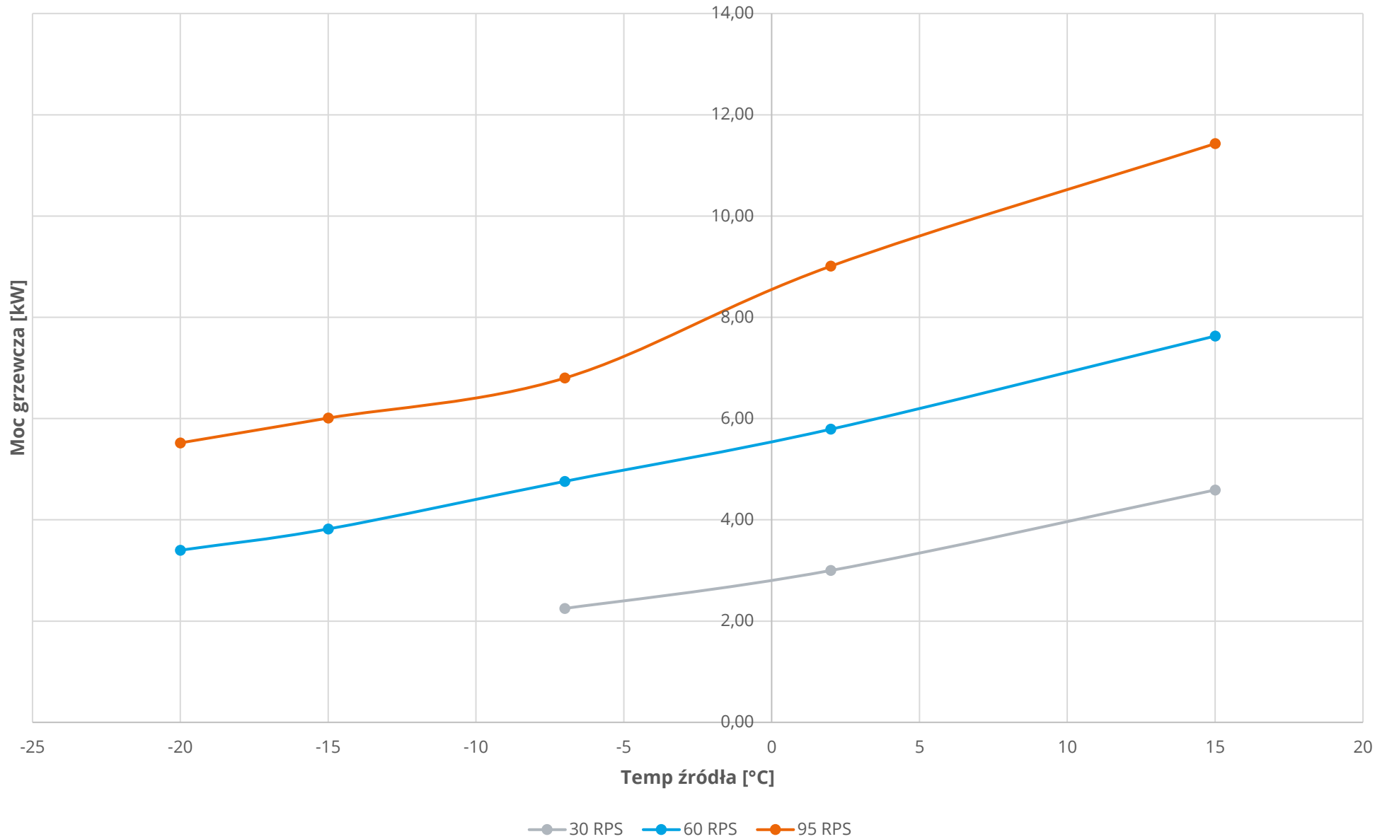
Wydajność ogrzewania pompa ciepła ZHHS-10K, Woda 30/35°
