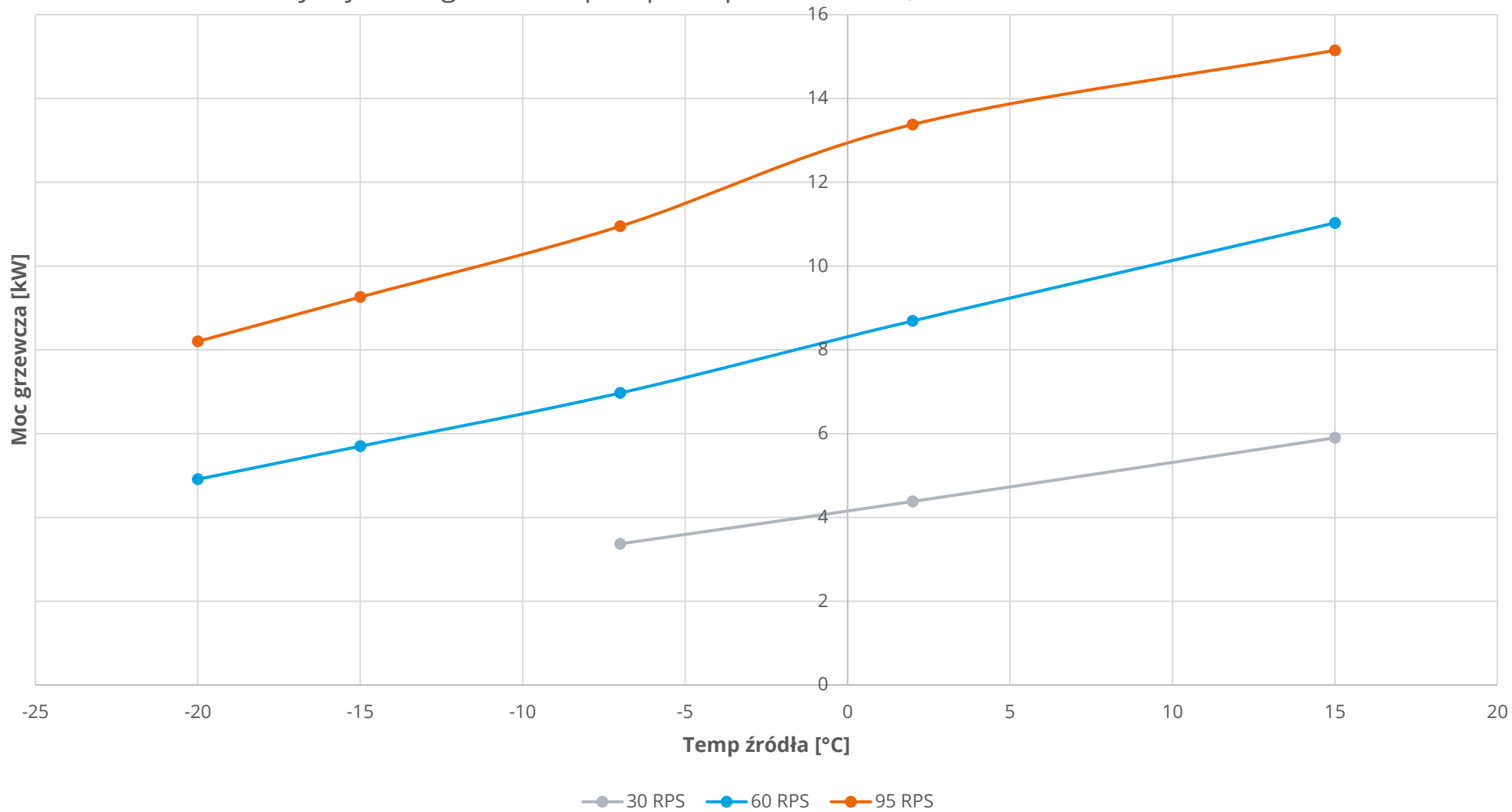
Wydajność ogrzewania pompa ciepła ZHHS-15K, Woda 47/55°C
